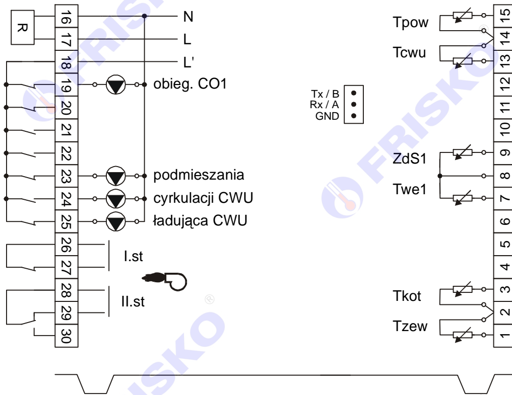
Schemat połączeń elektrycznych - układ U0 (montaż tablicowy - widok złącz na tylnej ścianie regulatora)
