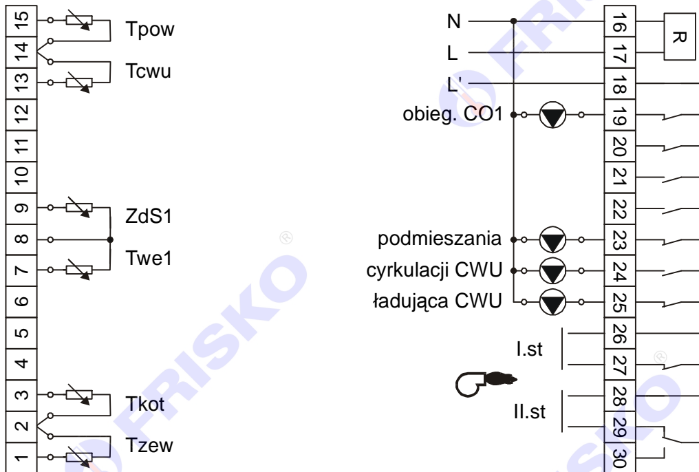
Schemat połączeń elektrycznych - układ U0 (montaż w cokole - widok złącz cokołu montażowego)
